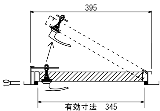
点検扉 亜鉛鉄板製内開き 型式一覧 (7種類)
