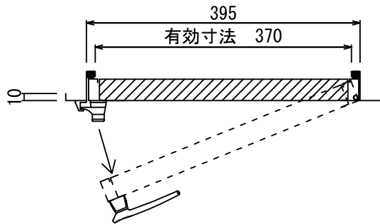
点検扉 ステンレス製外開き 型式一覧 (7種類)
