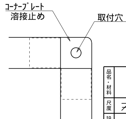
B部詳細
